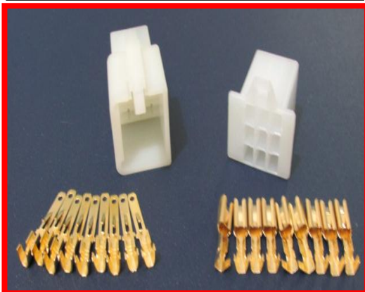
9 VIAS 1/8 COMPLETO (CON-9VH)
