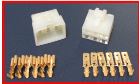
6 VIAS PIN T (CON-6VMP)
