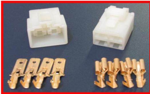
4 VIAS PIN T (CON-4VMP)
