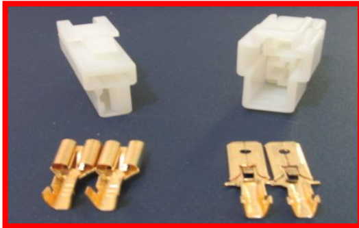
2 VIAS 1/4 COMPLETO (CON-2VH4)
