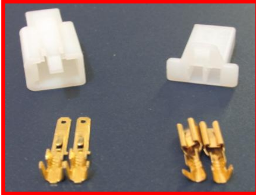
2 VIAS 1/8 COMPLETO (CON-2VH)
