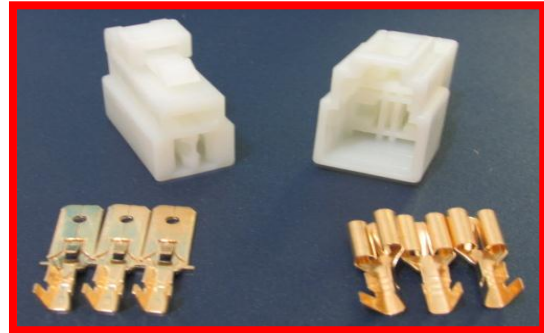
3 VIAS 1/4 COMPLETO (CON-3VH4)
